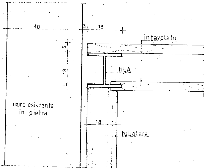
ARTICOLARE SOPPALCO
