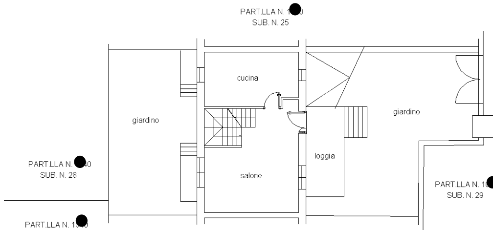
piano terra H. ml. 2.70
