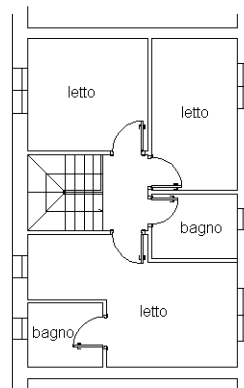
primo piano H. ml. 2.70
