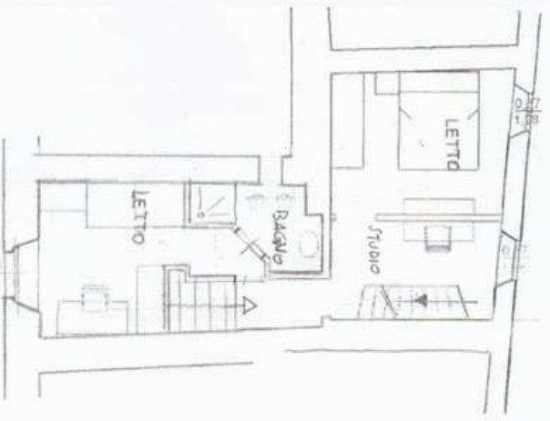
PIANO TERZO
