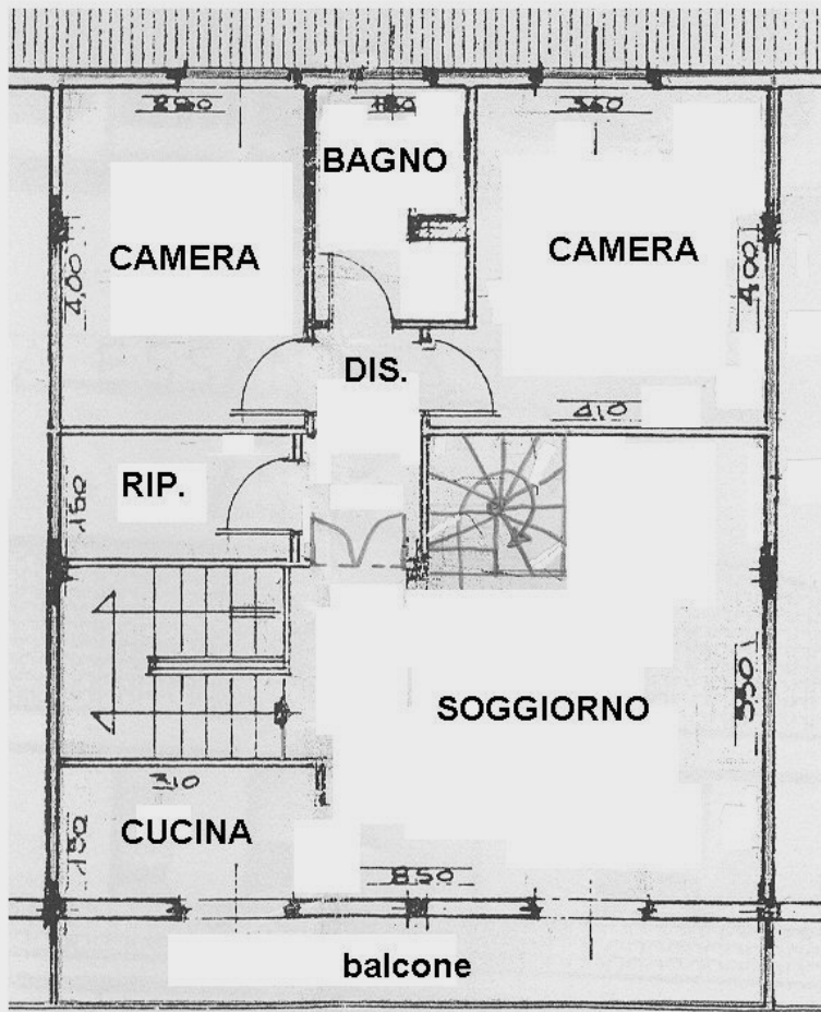
PIANO PRIMO
